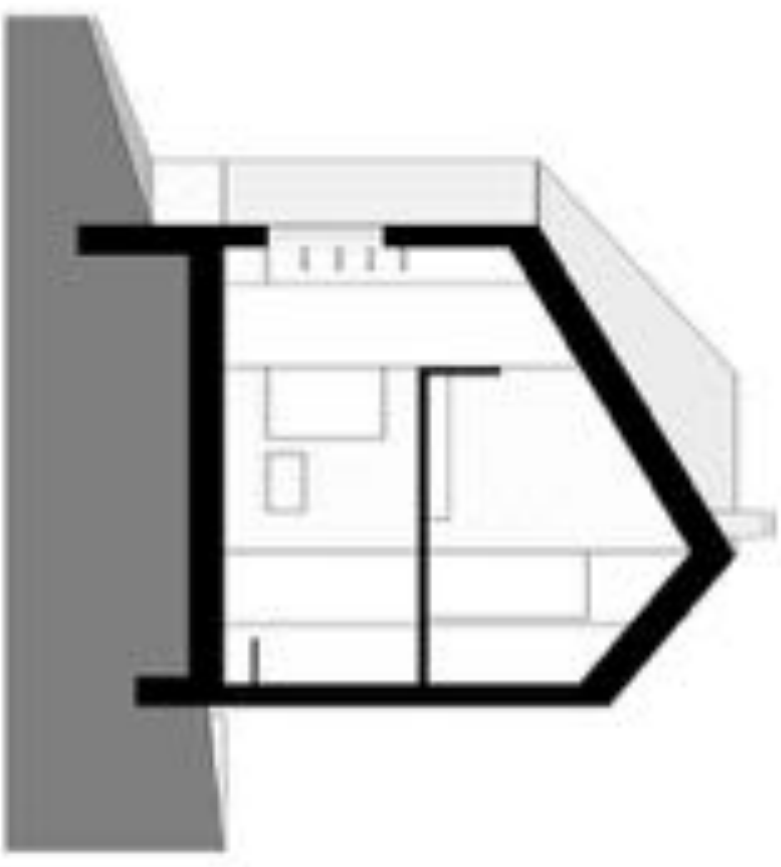
Schnitt 2 M 1:100
